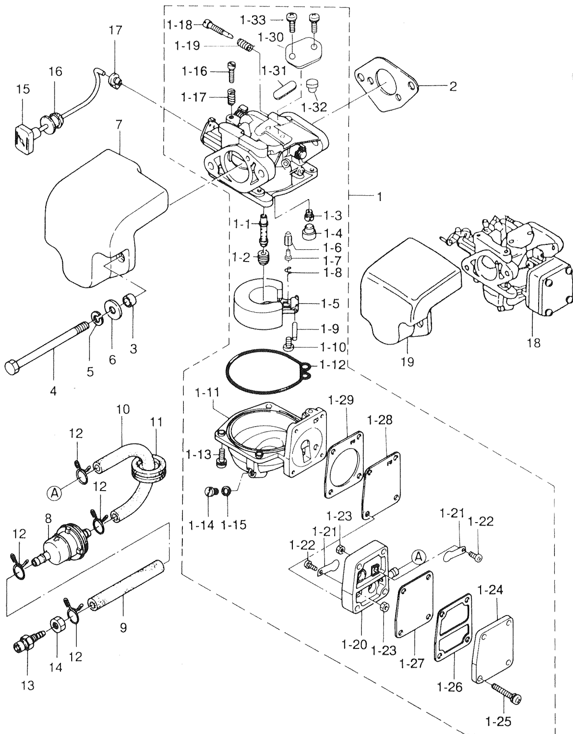
Fig. 4 キャブレタ CARUBRETOR
