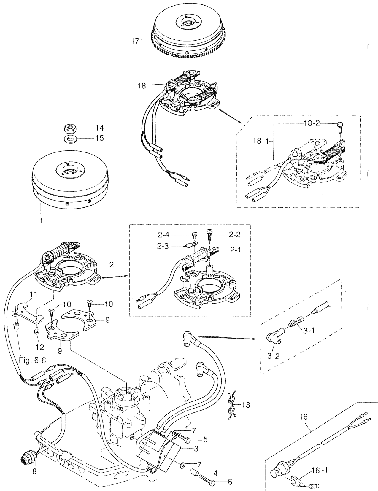
マグネト Fig. 5 MAGNETO
